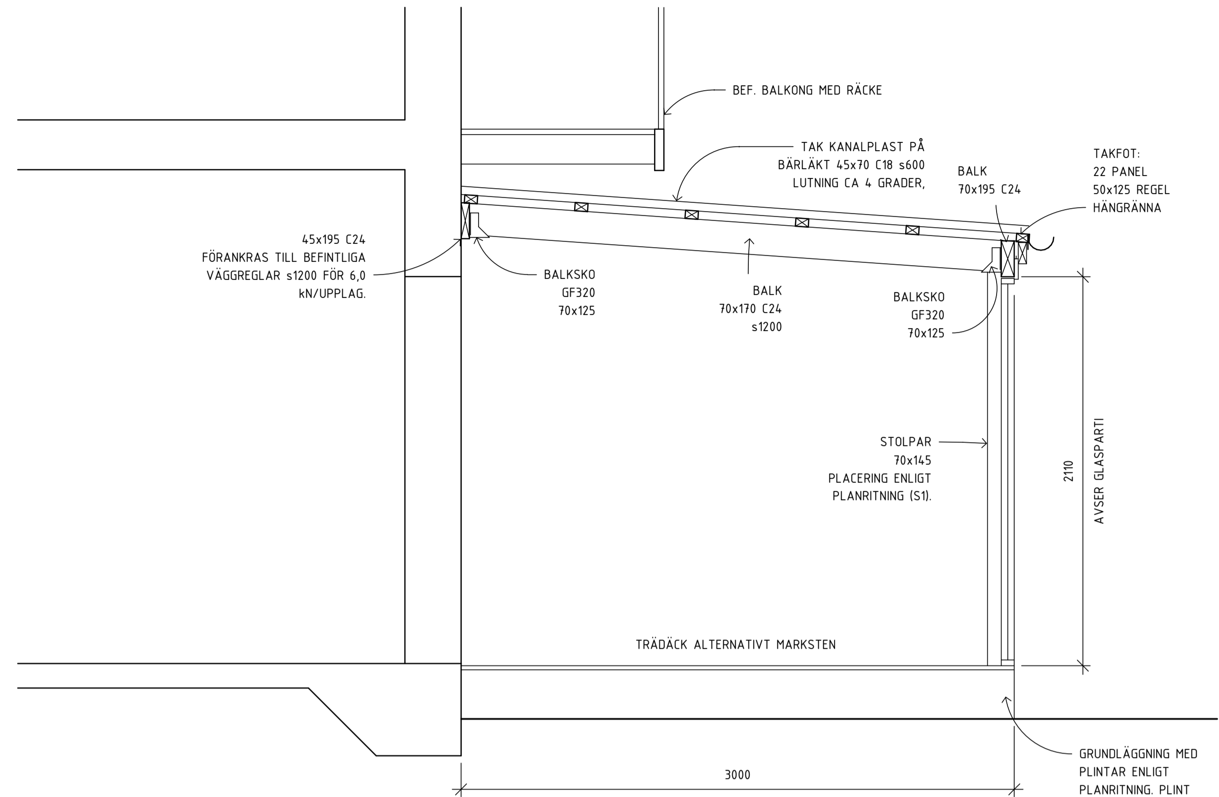
TEKNISK PRINCIPSEKTION 1:20
