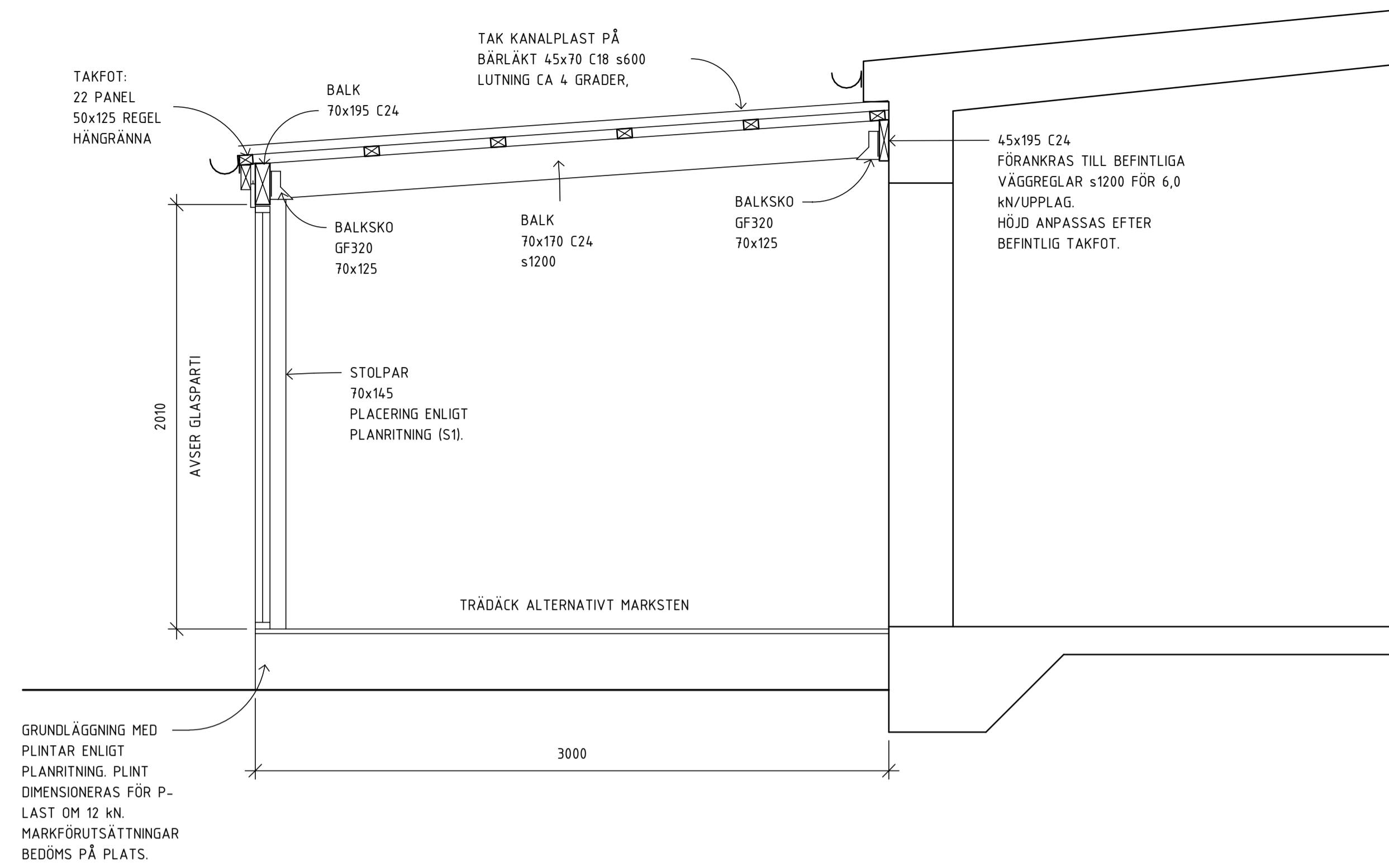
TEKNISK PRINCIPSEKTION 1:20
